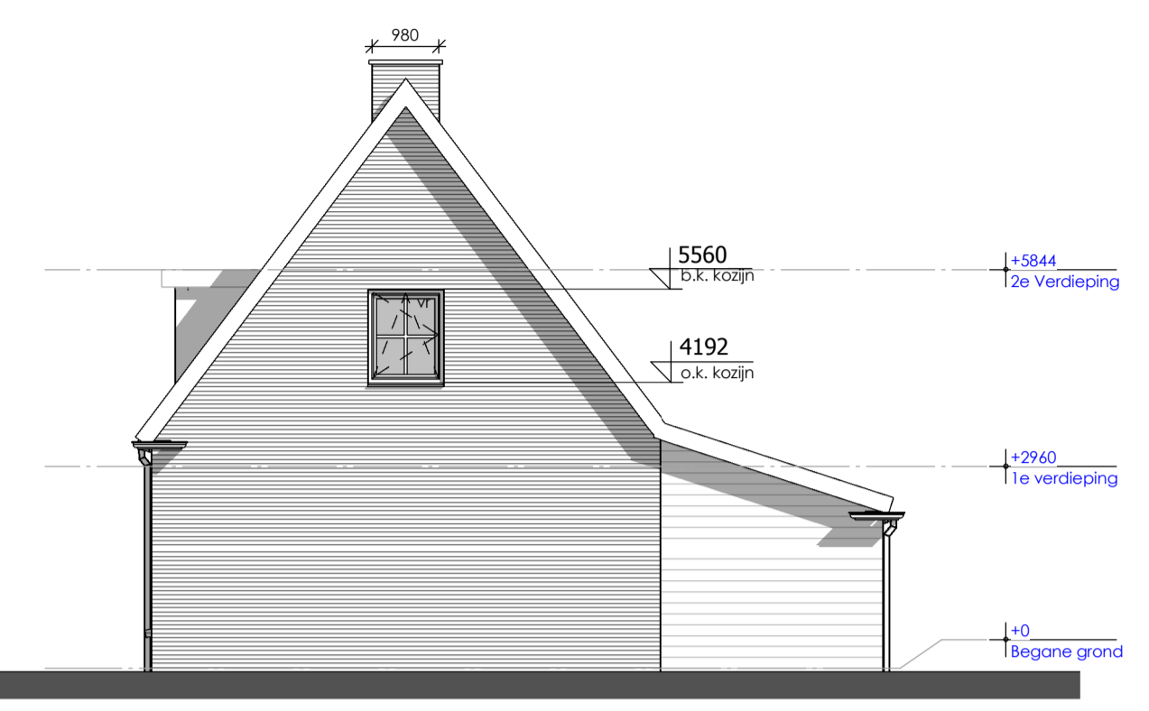
RECHTERZIJGEVEL
