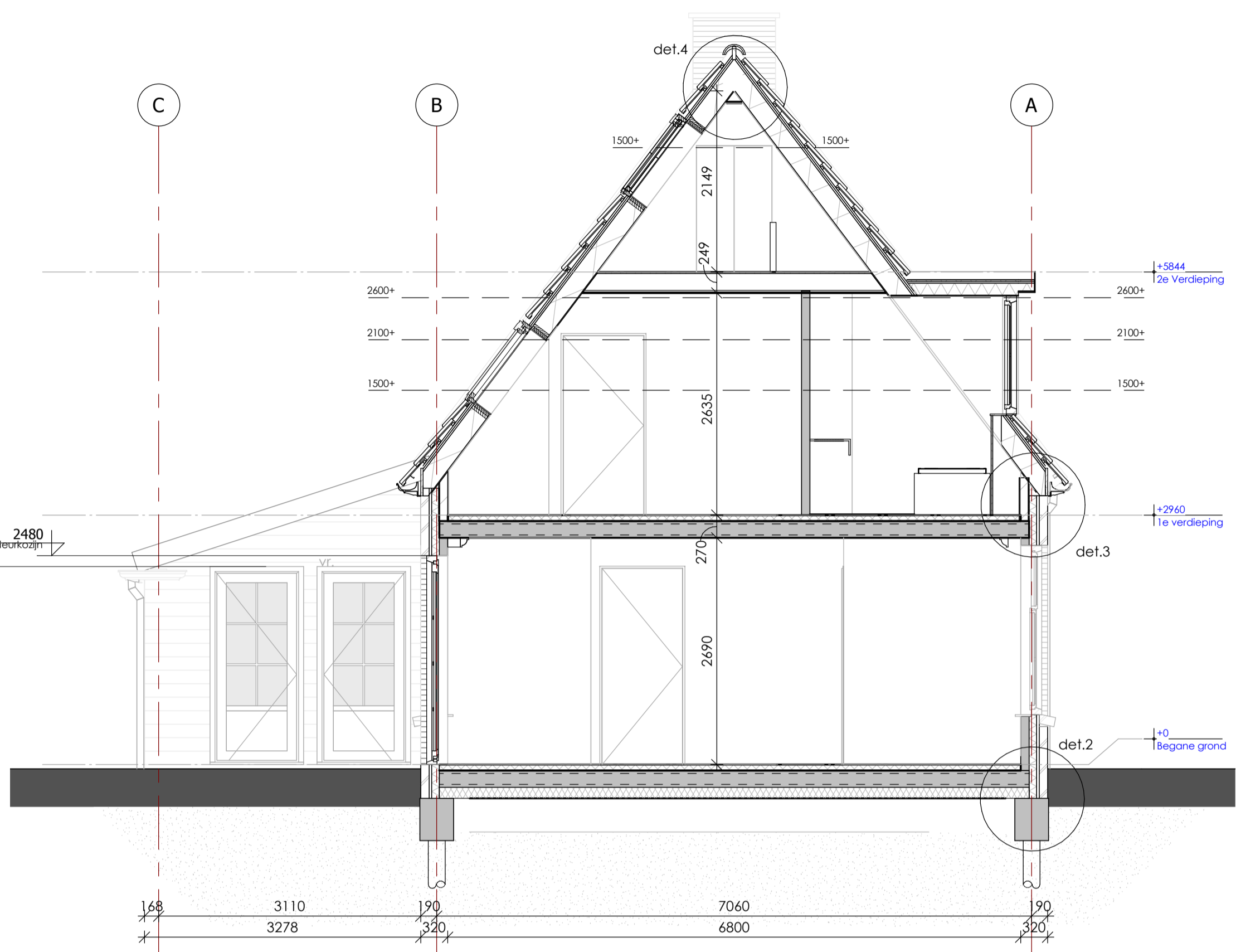
DOORSNEDE B-B
