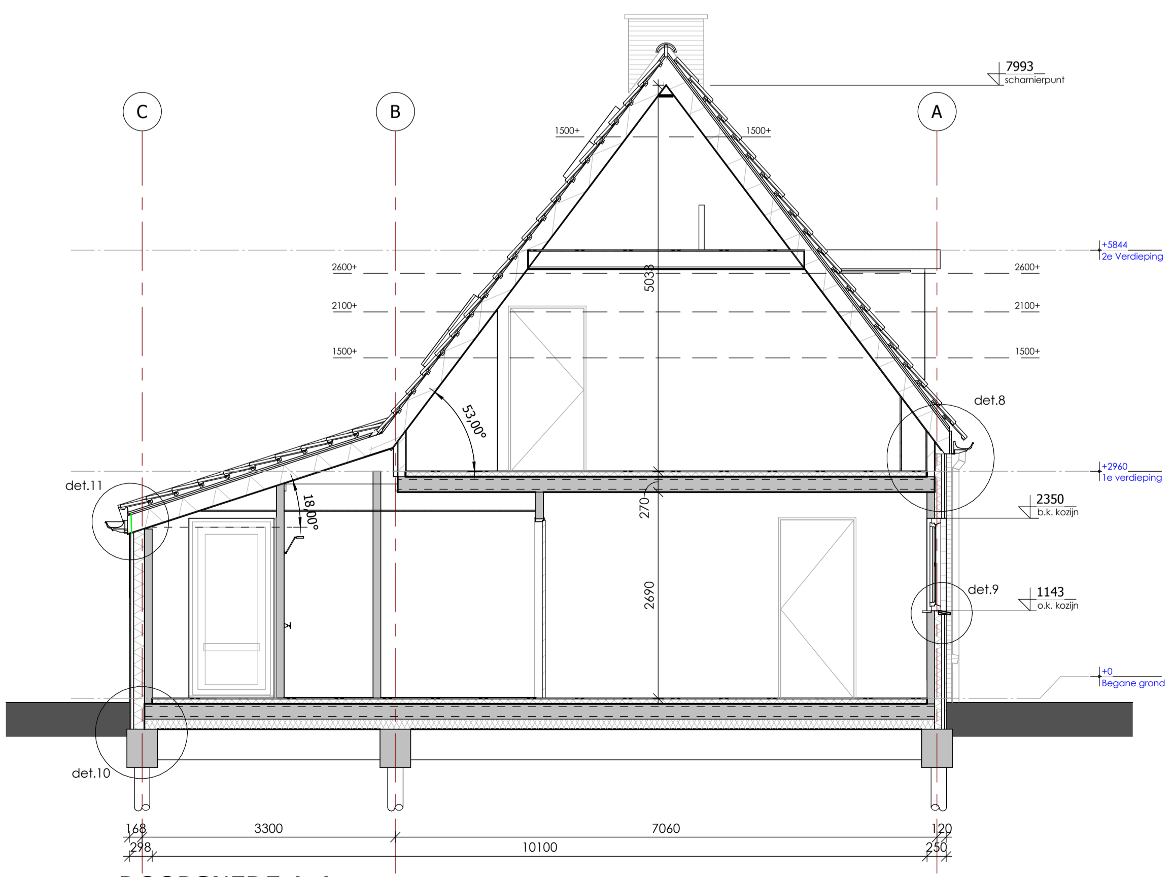
DOORSNEDE A-A
